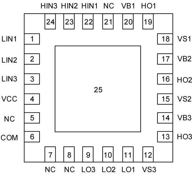
图 7-1 FD6288Q QFN24 顶视图
