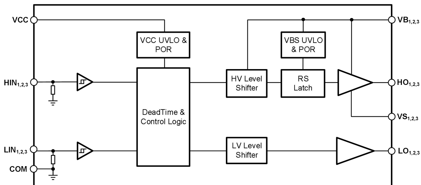
图 10-1 FD6288Q 功能框图
