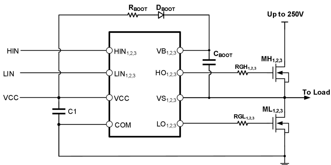
图 10-2 典型应用电路图
