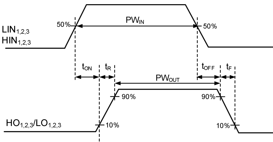
图 9-2 传输延时波形定义
