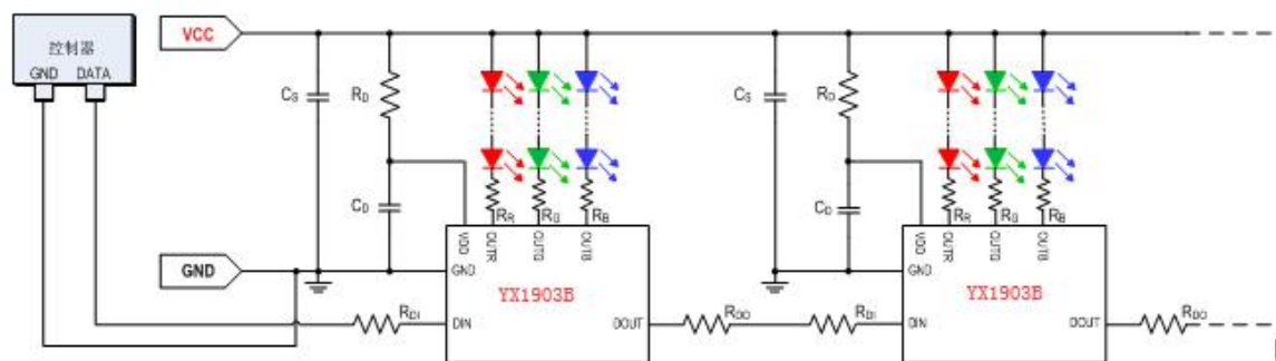
Fig. YX1903B 典型应用方案图
